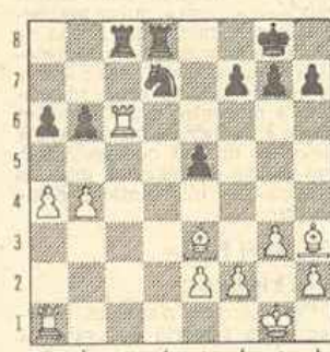
Après 24. Txc6!
