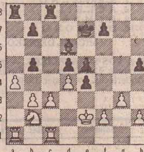
Après 21. ... e5!
