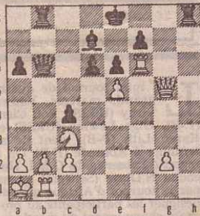
Après 25. e5!
